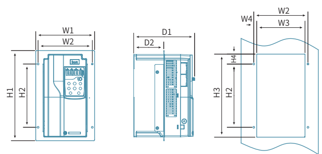
3-фазный 380 В перем. тока Схема фланцевого монтажа для модели 11~22 кВт
