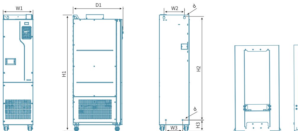
3-фазный 380 В перем. тока Схема установки для модели 220-630 кВт без выходного реактора
