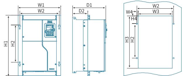
3-фазный 380 В перем. тока Схема фланцевого монтажа для модели 110~200 кВт
