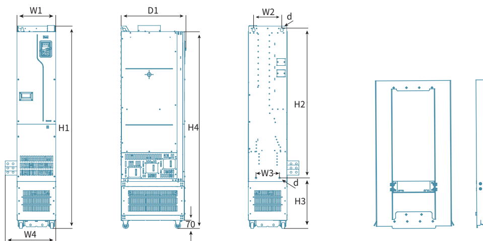
3-фазный 380 В перем. тока Схема установки для модели L3 220~630 кВт с выходным реактором
