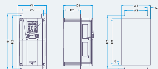
Фланцевый монтаж преобразователей 11 ~ 15кВт
