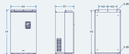
Настенный монтаж преобразователей 220 ~ 350кВт
