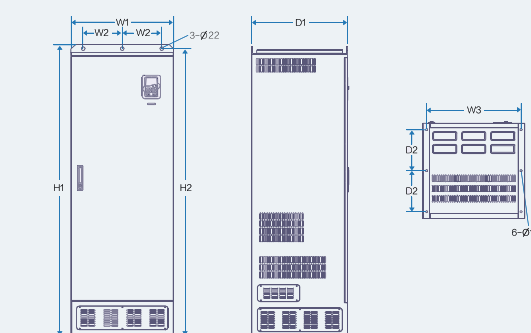
Напольный монтаж преобразователей 350—500кВт
