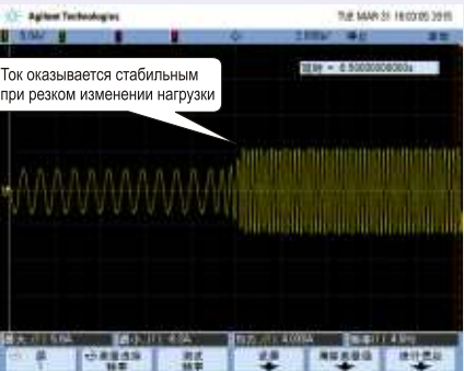
Форма тока при внезапной нагрузке в режиме векторного управления с полной нагрузкой на частоте 0,5 Гц.
