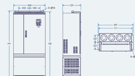
Напольный монтаж преобразователей 350—500кВт
