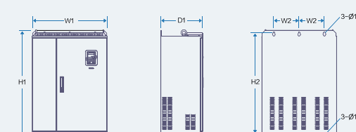
Настенный монтаж преобразователей 220 ~ 350кВт
