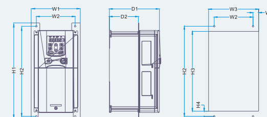
Фланцевый монтаж преобразователей 18,5 ~ 30кВт
