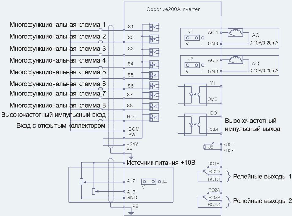
Схема подключения цепи управления
