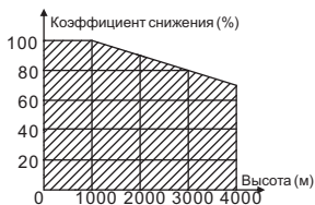
Рисунок 3-3. Снижение номинальной мощности преобразователя частоты GD20 в зависимости от высоты над уровнем моря.
