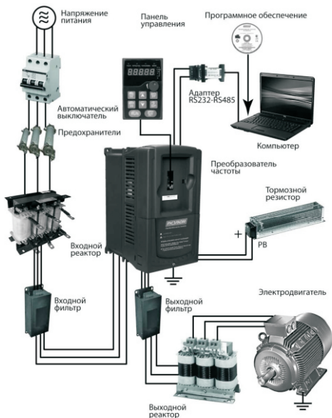
Рис. 12-1. Схема подключения дополнительного оборудования
